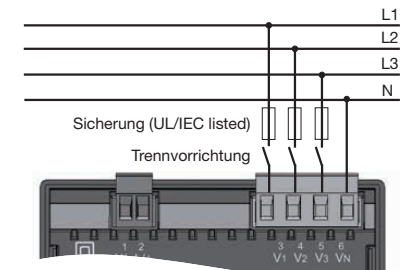
Anschlussvariante 3p 4w Spannungsmessung (Adr. 509 = 0, Standardeinstellung)
