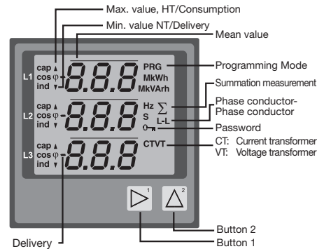
Fig. UMG 96 RM-EL display
