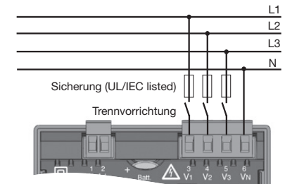
Anschlussvariante 3p 4w Spannungsmessung (Adr. 509 = 0, Standardeinstellung)
