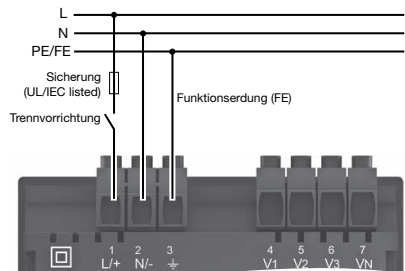
Abb. Anschluss Versorgungsspannung.
