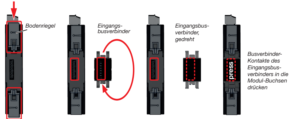
Abb.: Modul 800-CON - Rückansicht (mit Eingangsbusverbinder)
