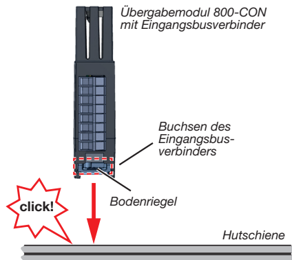
Abb.-Beispiel: Montage des Übergabemoduls mit Eingangsbusverbinder der räumlich entfernten Messstelle
