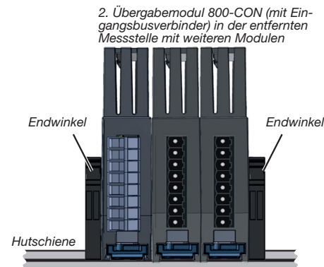
Abb.-Beispiel: Montage des Übergabemoduls mit Eingangsbusverbinder der räumlich entfernten Messstelle
